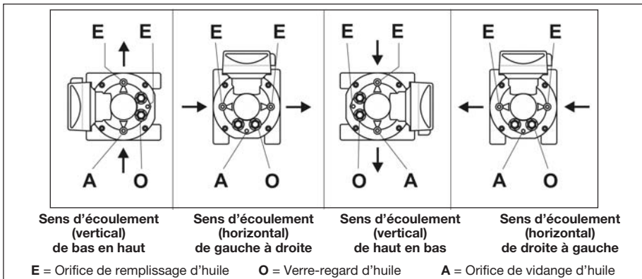
Fig. 6 : Positions d'utilisation admises, remplissage d'huile et indication du niveau d'huile (type RVG)
