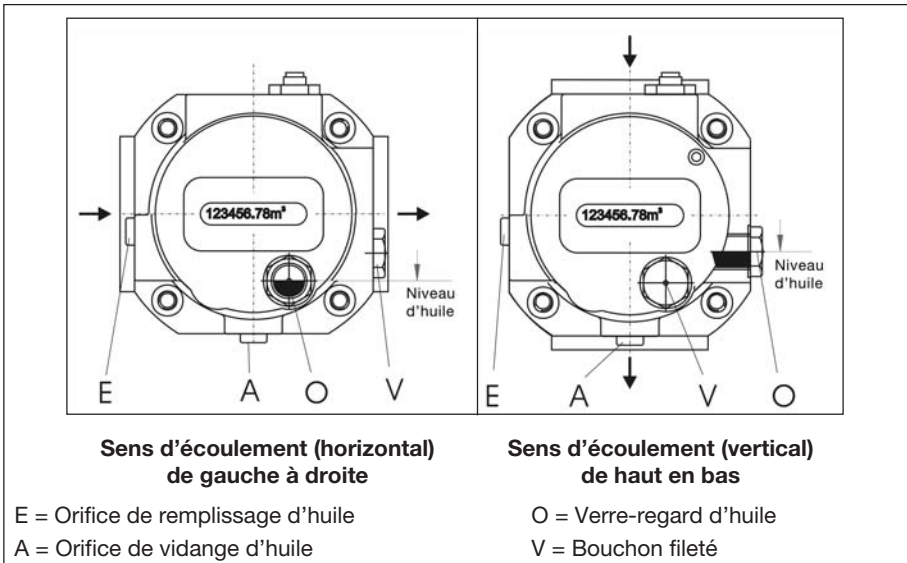
Fig. 7 : Position de montage horizontale et verticale, remplissage d'huile et indication du niveau d'huile ( type RVG-ST )
